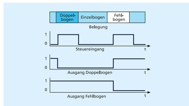
Trigger-Mode – pegelgesteuert
