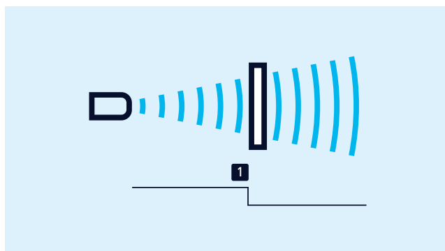
Teach-in для точки обнаружения (Метод A)
