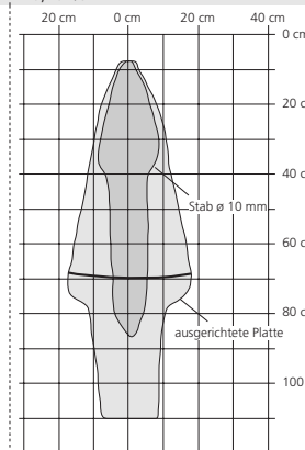
Abb. 5: Einstellung des Schaltpunktes bei unterschiedlicher Bewegungsrichtung des Objekts
