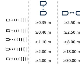
Fig. 1: Distances de montage, indiquant synchronisation/multiplex
