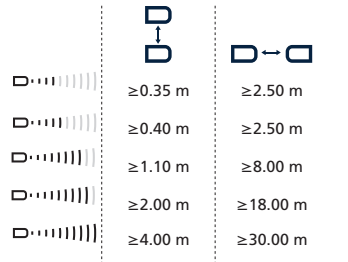
Fig. 1: Distances minimales de montage, indiquant synchronisation/multiplex
