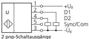
2 pnp-Schaltausgänge
