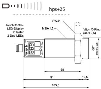
1 pnp-Schaltausgang + Analogausgang
