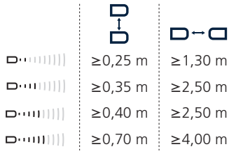
Abb. 2: Montageabstände, unterhalb derer Synchronisation genutzt werden sollte
