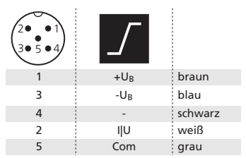
Abb. 1: Pin-Belegung mit Sicht auf den Sensor-Stecker und Farb-Kodierung der microsonic-Anschlusskabel
