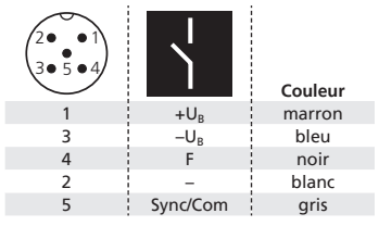
Fig. 2: Attribution des broches avec vue sur la prise du capteur et codage de couleur du câble de connexion microsonic
