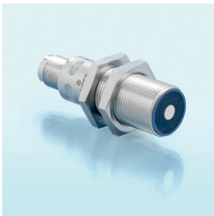
ipc+15/CFF Ultraschall-Näherungsschalter mit einem Push-Pull-Schaltausgang und IO-Link-Schnittstelle
