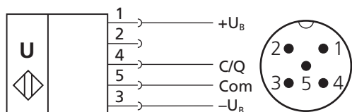
Bild 3: Anschlussbild des crm+ Sensors
