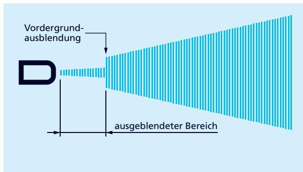
Bild 11: Messkonfiguration – Vordergrundausbldung
