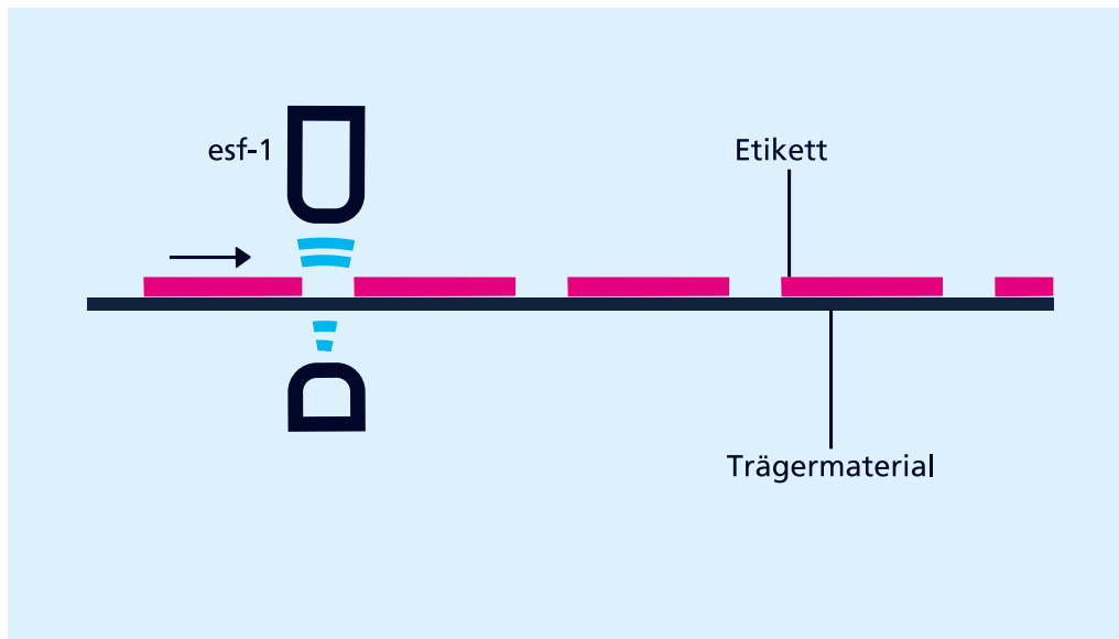
esf-1 als Etikettensensor
