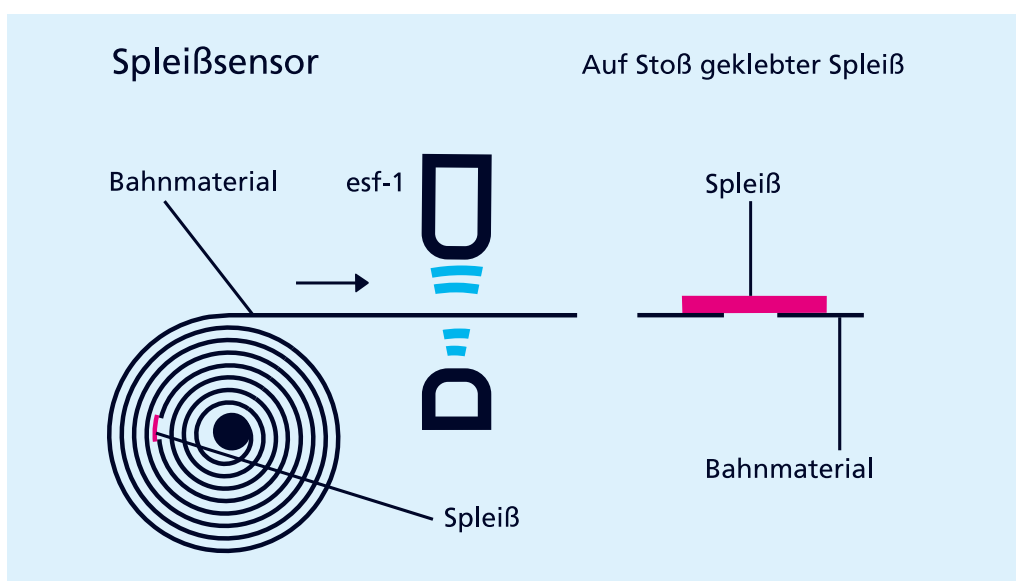
esf-1 als Spleißsensor
