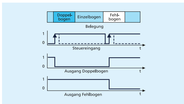
Trigger-Mode – flankengesteuert
