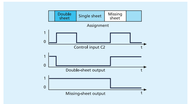
Trigger-mode – niveaugestuurd
