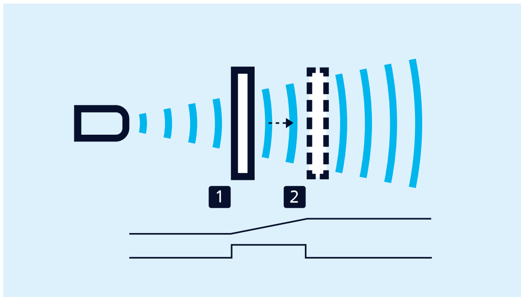
Teach-in van een analoge karakteristiek of van een venster met twee schakelpunten
