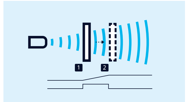
Teach-in и график настройки диапазона для аналогового выхода или для 2-х зон переключения
